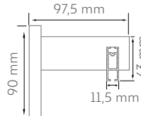
Riel Urban doble
