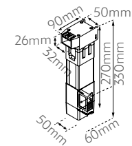
Motor Riel XXL a techo para LYNX
