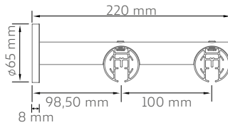
Riel Aeris doble
