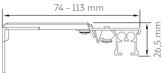
Ondas Perfectas cordón a techo
