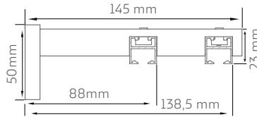
Riel Square doble
