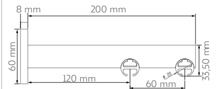
Riel Dike doble
