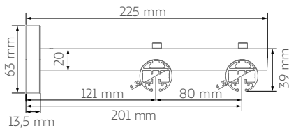
Riel Elpis doble
