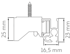
Riel Elementos techo
