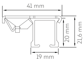
Ondas Perfectas bastón a techo
