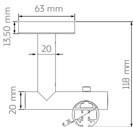
Riel Elpis a techo
