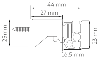
Riel Elementos techo
