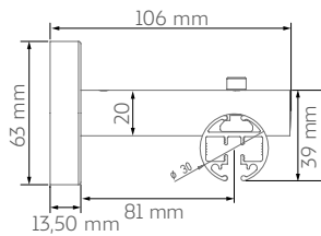
Riel Elpis a pared
