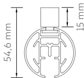
Riel Aeris a techo
